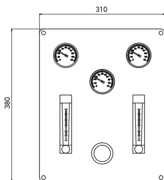
图 14 LZB-( ) DK/2/M/RA/8/P
