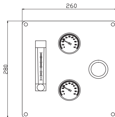
图 13 LZB-( ) DK/1/M/RA/8/P
