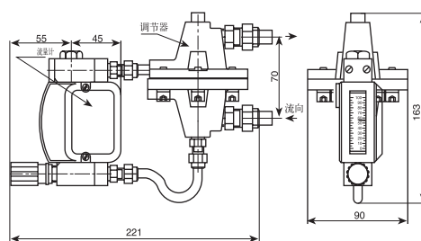
图 10 LZWB/D/RA/8/P
