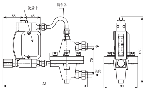
图 9 LZWB/D/RE/8/P
