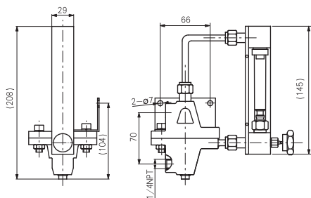
图 7 LZB-( ) DK/D/RE/8/P
