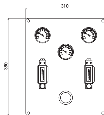
图 16 LZWB/2/M/RA/8/P
