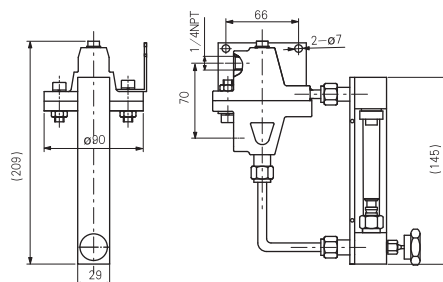
图 8 LZB-( ) DK/D/RA/8/P
